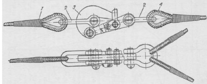
Рис. 2.. Крепление буксирного троса к браге (узел Л):
