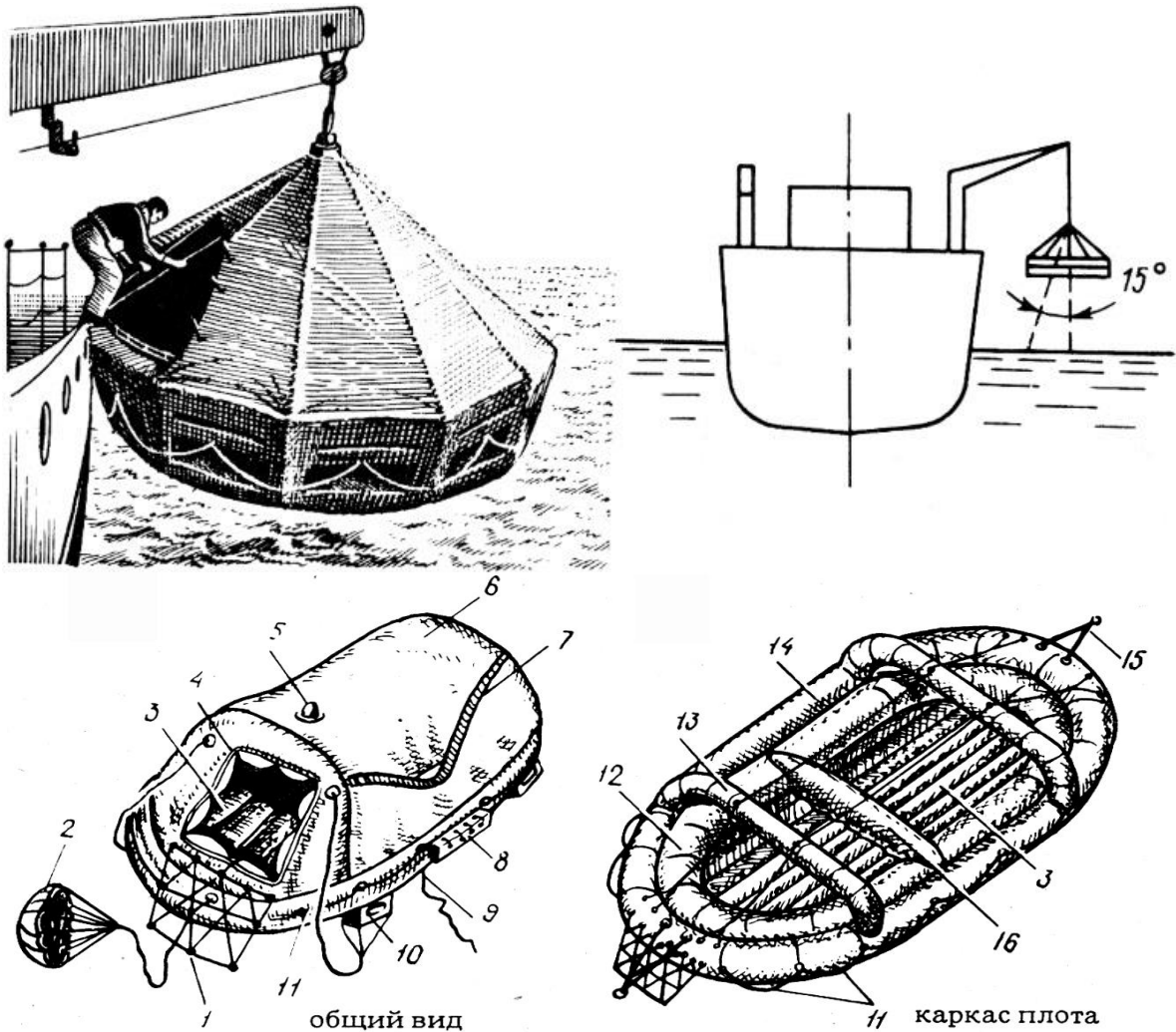
Спасательный надувной плот
