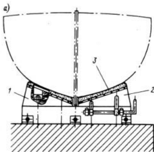
разрез закрытой моторной шлюпки
