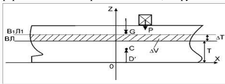
Рис. 6. Изменение остойчивости судна от приема или снятия (расходования) грузов. Метацентрическая высота, характеризующая остойчивость судна, вследствие всех названных причин, получит следующее изменение:
