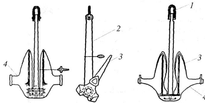
Рис. 9-4. Якорь Матросова:
