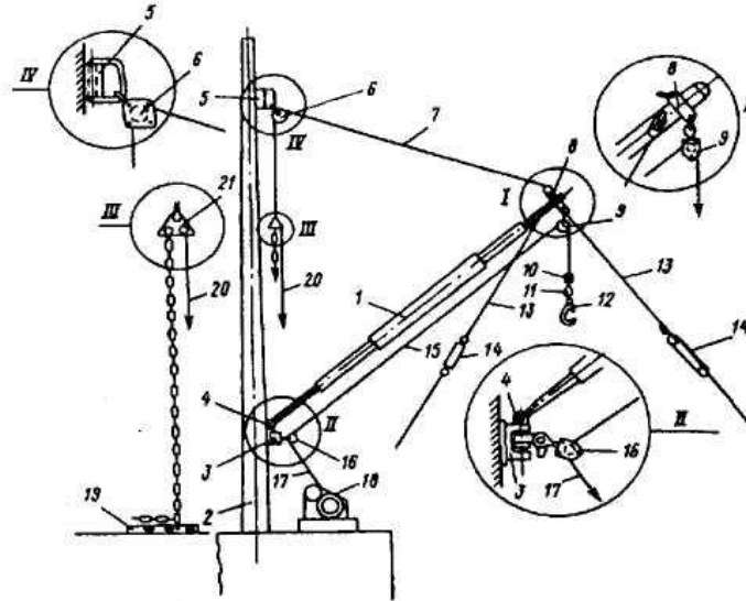
Рис. 5.18. Грузовая стрела:
