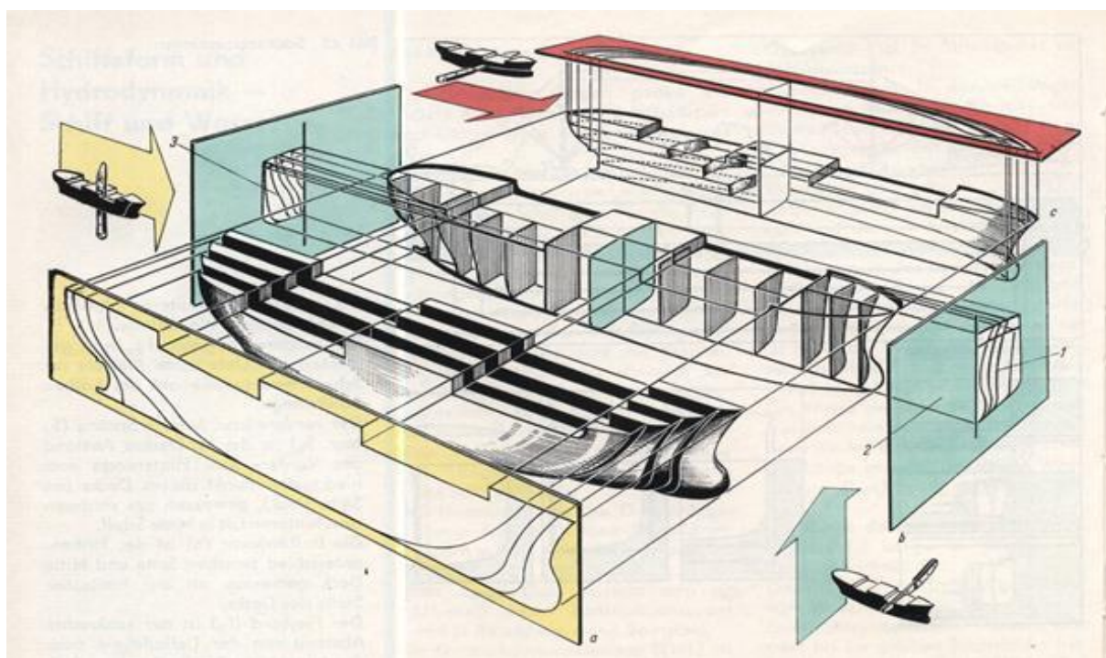
Рис. 16. Изображение корпуса судна на теоретическом чертеже: a — бок; b — корпус; c — полуширота; 1 — корпус носовой оконечности; 2 — диаметральной плоскости; 3 — корпус кормовой оконечности
