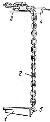
Рис. 9-6. Крепление якорной цепи к корпусу судна с помощью живака-галса: 1 - кильсон; 2 - живака-галсовый конец; 3 - глаголь-гак; 4 - палубный клюз; 5 – обух Стопоры служат для удержания якорной цепи в необходимом положении. Устанавливаются на палубе между шпильем (брашпилем) и якорным клюзом (рис. 9-7).
