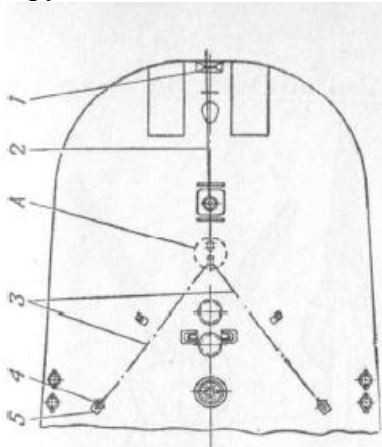
Рис.1. Буксирное устройство судна:
